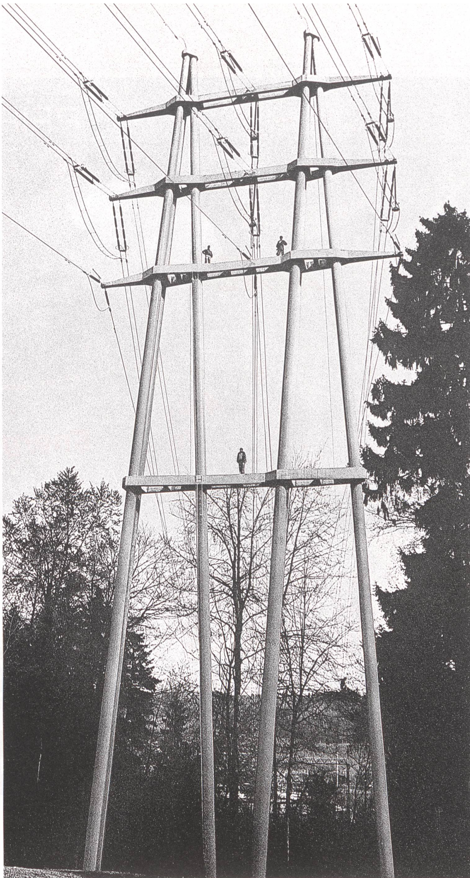
380/220/110 KV-Leitung Hellbühl – Littau
