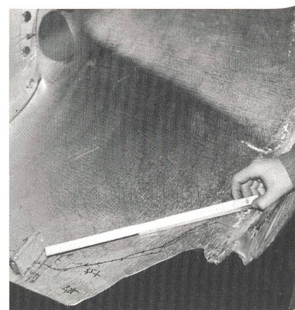
Fig. 2 Etat des pales après six ans d'exploitation
