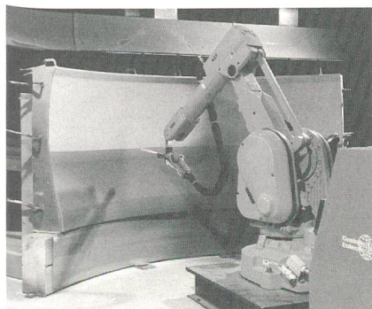
Fig. 6 Revêtement d'un élément de manteau de turbine
