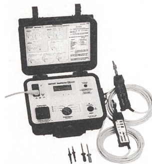
Multitester 9032 für Anlagen, Maschinen und mobile Geräte
