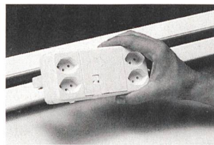
Brüstungskanal-Stromschiene KB-System
