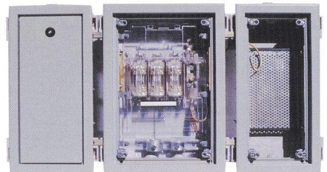
Unterputzkasten ENC / TV / TT
