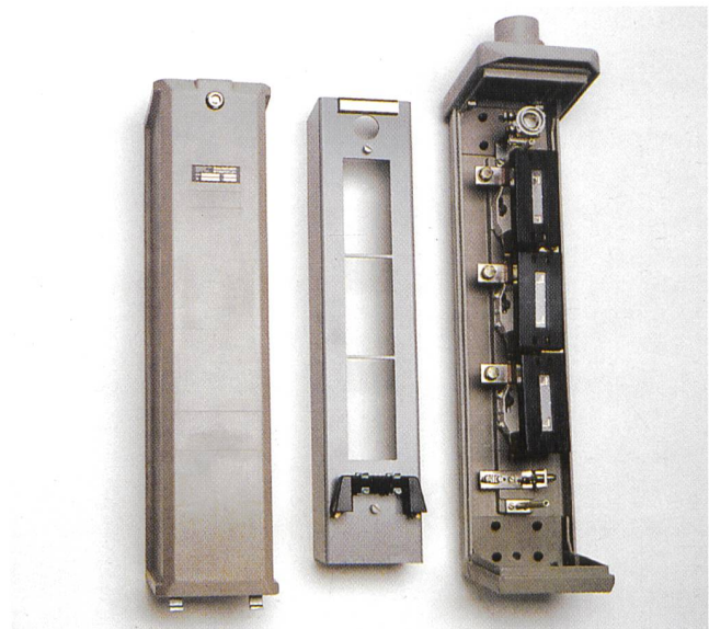
Strangsicherungskasten mit diversen Einbaumöglichkeiten
