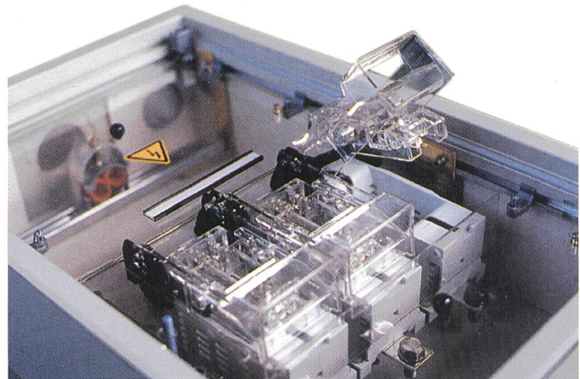
Anschlusskasten mit Sicherungselement LTS-400/S
