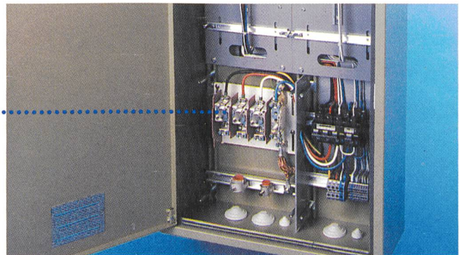
Platine mit Diazed- oder DIN 00-Elementen
