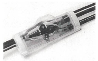
Parallelabzweigmuffe HME-A-150
