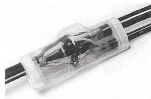
Parallelabzweigmuffe HME-A-150
