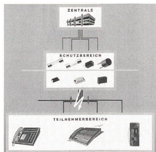
Stromimpulsfeste Sicherungseinsätze
