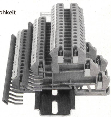
Initiatorenklemmen mit Verbindungsrechen
