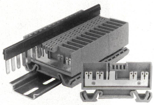
Flachsteckerklemmen mit Verbindungsrechen
