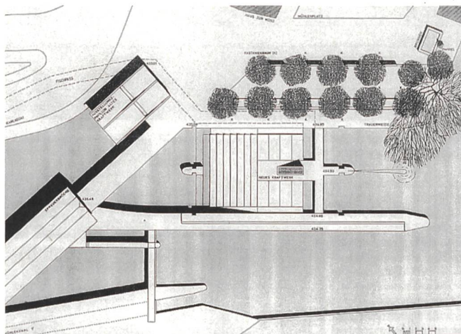
Bild 3 Grundriss des neuen Wasserkraftwerks: bei extremen Hochwasserphasen überflutet.
