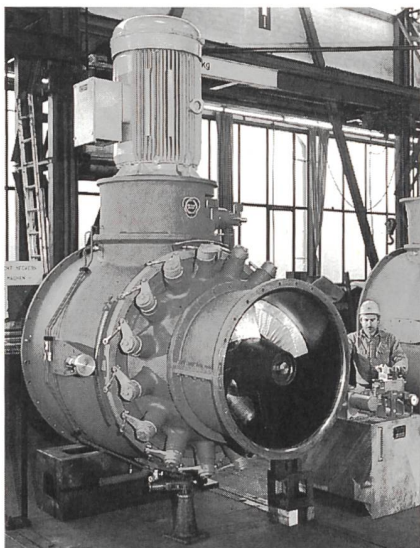
Bild 2 Kegelrad-Rohrturbine: kompakt und geräuscharm.
