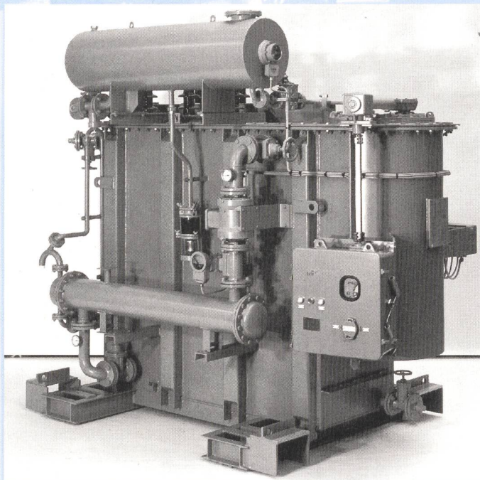
5 MVA Reguliertransformator, wassergekühlt, ausgeführt für die Kraftwerke Oberhasli, Innertkirchen / BE
