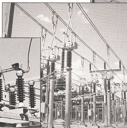
Scherentrenner 72,5–420 kV
