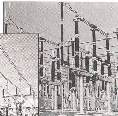
Drehtrenner: 170–420 kV
