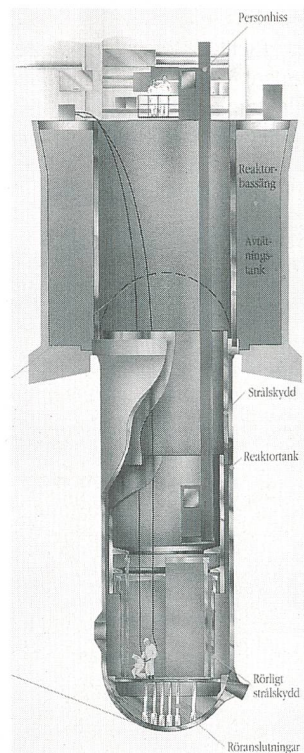
Aussergewöhnliche Arbeiten im Reaktordruckbehälter: dazu wurden unter anderem Strahlschutzzyliner und ein spezieller Personenaufzug eingebaut
