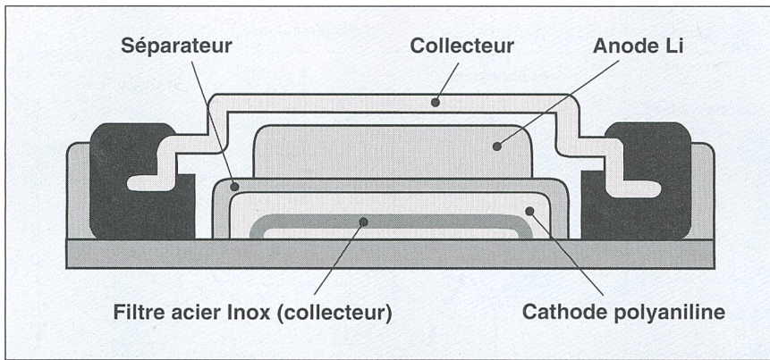
Figure 7 Coupe d'une pile bouton lithium/polyaniline
