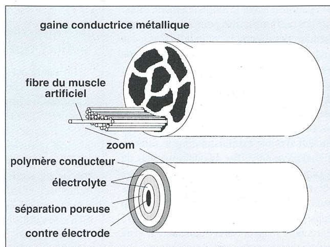
Figure 15 Actuateur électromécanique semblable à un muscle naturel
