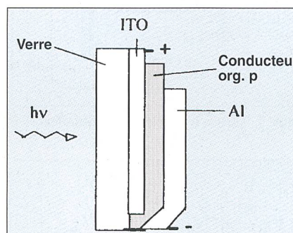
Figure 10 Structure d'une cellule photovoltaïque organique Schottky
