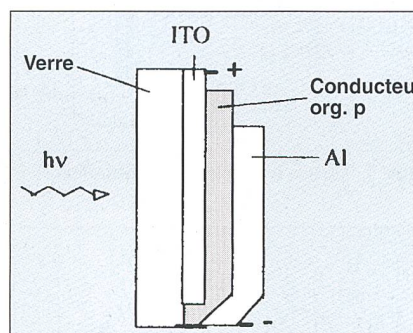
Figure 10 Structure d'une cellule photovoltaïque organique Schottky
