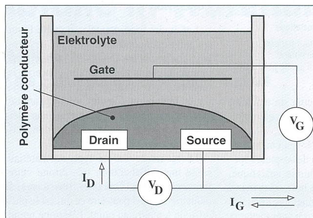
Figure 13 Représentation schématisée d'un capteur électrochimique
