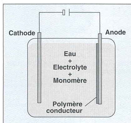
Figure 5 Schéma d'une électropolymérisation
