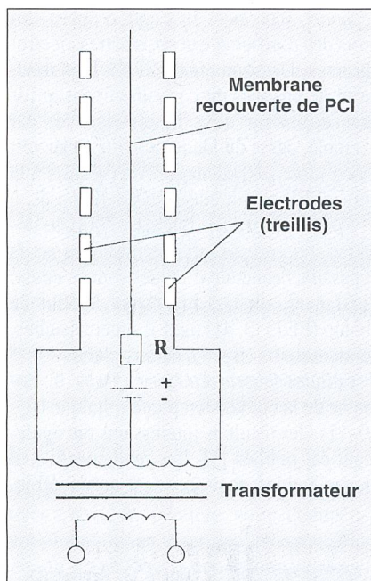
Figure 16 Haut-parleur électrostatique Illustration schématique d'un haut-parleur électrostatique utilisant une membrane avec 0,1 \mu\text{m} de polyaniline sur 6 \mu\text{m} de polyester
