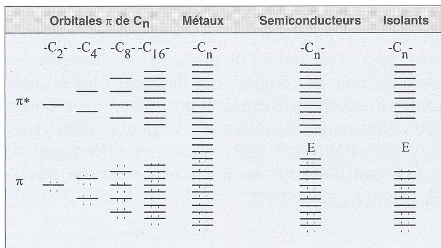
Figure 2 Diagramme des bandes d'énergie pour des polyènes de grandeur croissante
