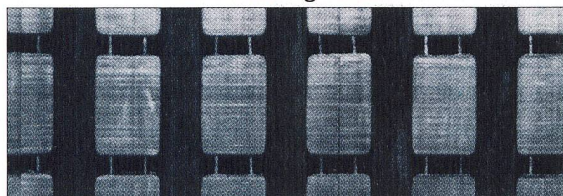
Magnetkreis nach der Reinigung durch Maiskolbengranulat
