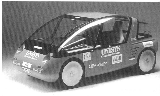
Das Horlacher «Weltrekord-Leichtelektromobil» – eine Weiterentwicklung wird in Bern ausgestellt sein
