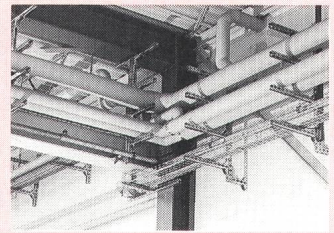
Universelles Befestigungssystem Multifix
