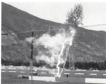
Internationale 380-kV-Kurzschlussversuche: Wie reagieren die Schutzrichtungen auf einen Baum im Erdschluss?
