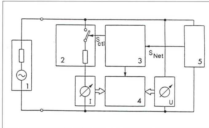
Figure 4 Schéma-bloc du système de mesure
