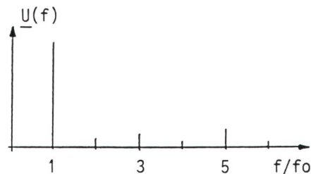
Figure 3 Exemple du spectre de la tension du réseau
