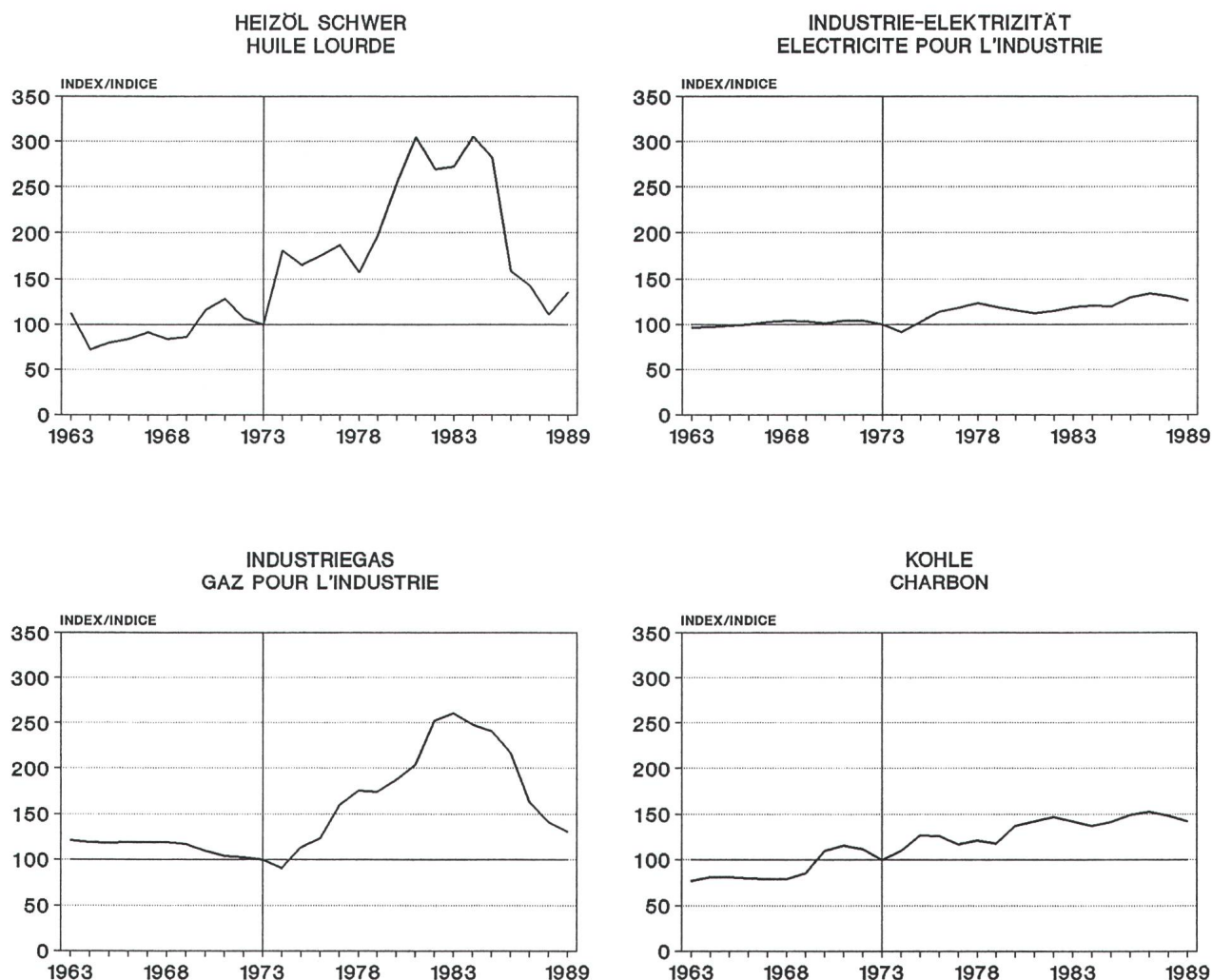
Fig. 11 Preisentwicklung auf der Grosshandelsstufe (Grosshandelspreise real)
