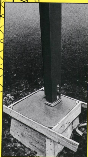
Sanierung von Mastsockeln
