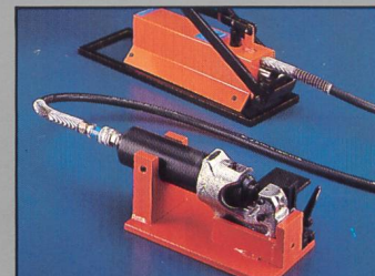
PNEUMATISCHES STANZ- WERKZEUG zum Stanzen von lamellierten Stromschienen.
