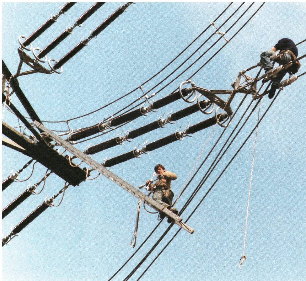
Spannschloss: unfallsicher dank offener Bauweise mit visueller Kontrollmöglichkeit des Montagevorganges.
