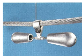
Schwingungsdämpfer: ausgeglichene Leistungs-Charakteristik; wirksam über breites Frequenz-Spektrum.
