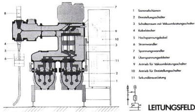
Metallgekapselte, SF 6 -isolierte Mittelspannungsschaltanlage PG 100 mit Vakuumleistungsschaltern, für 12/24/36 kV. Schnitt durch Doppelsammelschienen-Leitungsfeld.
