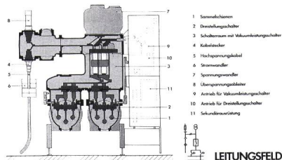
Metallegekapselte, SF 6 -isolierte Mittelspannungsschaltanlage PG 100 mit Vakuumleistungsschaltern, für 12/24/36 kV. Schnitt durch Doppelsammelschienen-Leitungsfeld.
