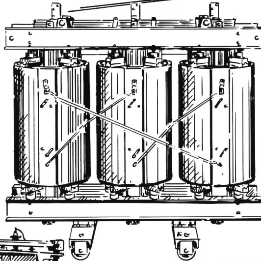
GISSHARZ- TRANSFORMATOREN
