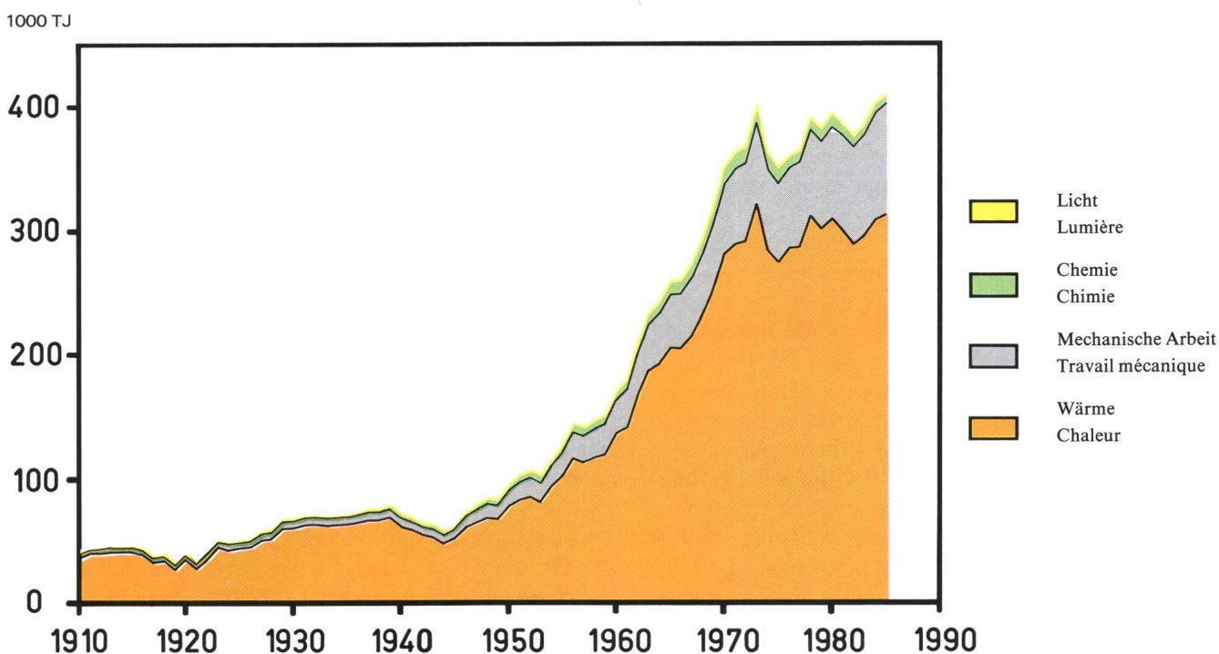
Fig. 13 Nutzenergie: Aufteilung auf die Anwendungsgebiete Energie utile: Ventilation par types d'utilisation
