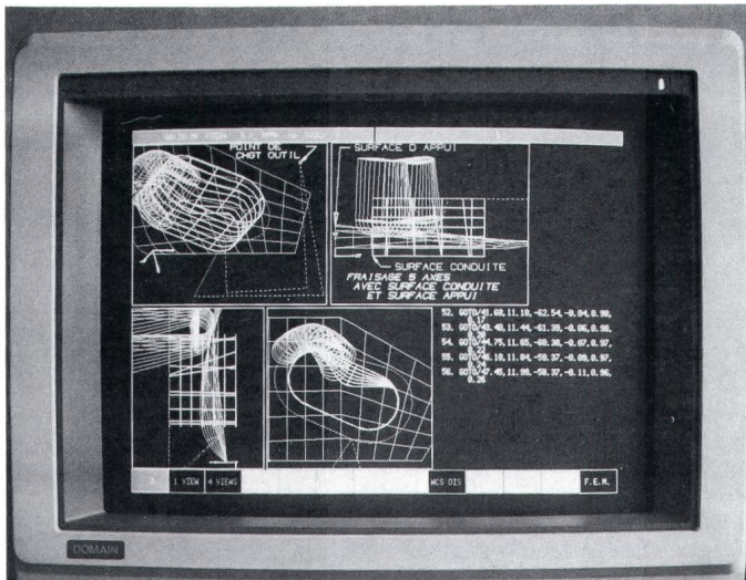
Figur 1 Sachsige NC-Bearbeitung am Auto-trol
