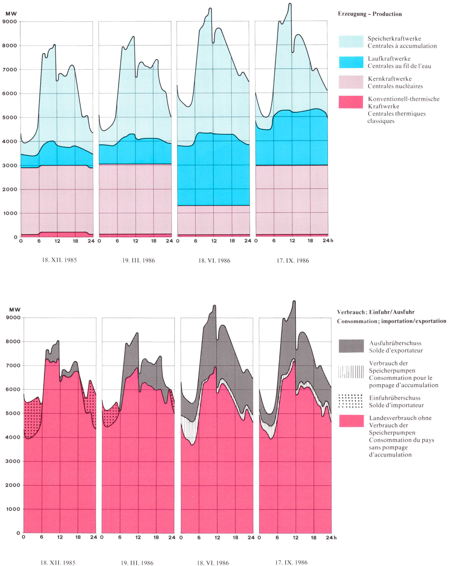
Fig. 12 Belastungsverlauf am 3. Mittwoch des Monats: Erzeugung (oben) - Verbrauch (unten)
