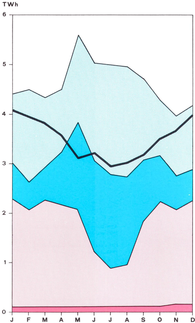
Fig. 4 Monatliche Erzeugungsanteile und Endverbrauch im Kalenderjahr 1986
