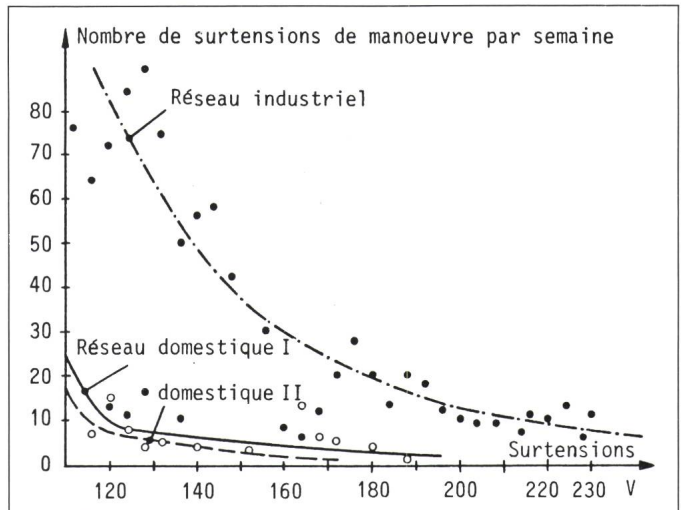
Fig. 2 Statistique des surtensions de manœuvre d'une durée de 0,5 à 800 \mu s
