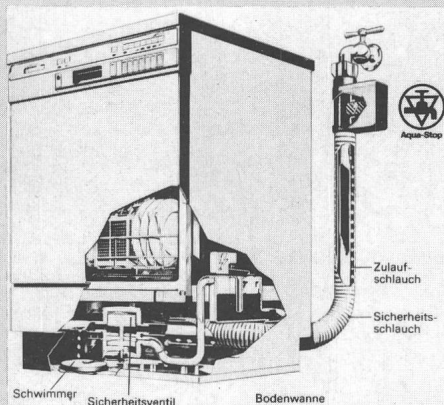
Aque-Stop Sicherheitssystem für Geschirrspüler
