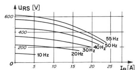
Fig. 9 Tension composée en fonction du courant de charge avec la fréquence comme paramètre et \cos \varphi = 1
