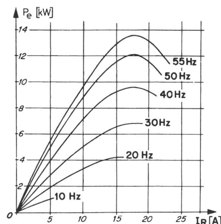
Fig. 8 Puissance électrique P_e du générateur en fonction du courant de charge avec la fréquence comme paramètre et \cos \varphi = 1
