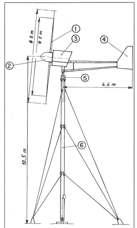
Fig. 1 Aérogénérateur FMN de 5 kW
