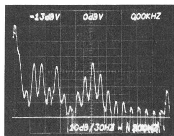
Fig. 12 Spectre de tension résultant du courant soutiré à 1025 Hz 1025 U_{eff} = 20 mV
