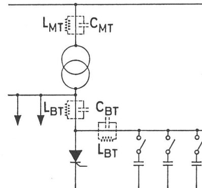
Fig. 5 Schéma simplifié d'un réseau de distribution avec convertisseur statique et compensation d'énergie réactive
