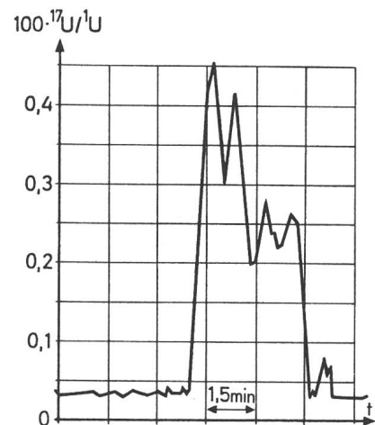
Fig. 1 Accroissement d'une tension harmonique de rang 17 durant le démarrage d'un convertisseur statique de 250 kW
