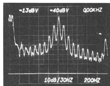
Fig. 11 Spectre d'un courant harmonique soutiré du réseau, centré sur 1025 Hz Echelles: 200 Hz/div; 10 dB/div; 1025 I_{eff} = 0,16 A
