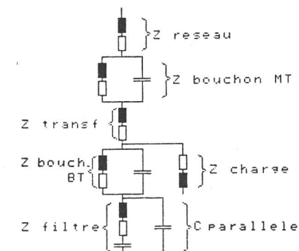
Fig. 6 Schéma équivalent correspondant au réseau de la figure 5
