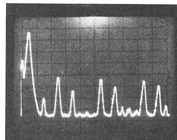
Fig. 10 Spectre de tension d'un réseau monophasé alimentant des convertisseurs statiques Echelles: 100 Hz/div; 10 dB/div; U_1 = 220 V
