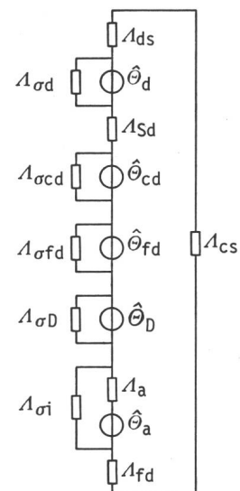
Fig. 2 Schéma magnétique équivalent d'un pôle (axe direct)
