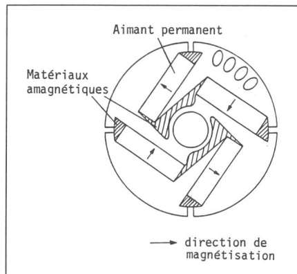
Fig. 5 Coupe de principe d'un moteur du type Siemossyn
