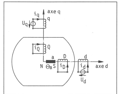
Fig. 6 Circuit électrique équivalent du moteur Siemossyn
