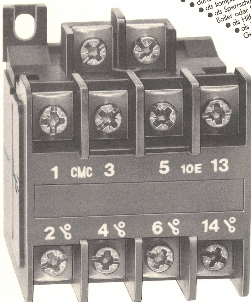
Originalgrösse 45 × 58 × 52 mm
