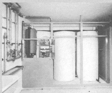
Wasser-Zentralspeicher-Kleinbehälteranlage
