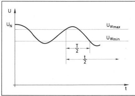
Fig. 2 Délestage d'après l'oscillation de la tension
