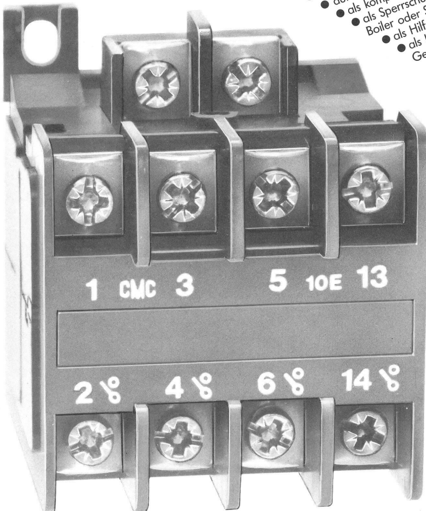
Originalgrösse 45 × 58 × 52 mm
