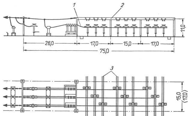
Fig. 6 220-kV-Freiluftschaltanlage in halbhoher Bauweise mit Einsäulentrennern und Sammelschienen oben, sog. Diagonalbauform [A 4]
