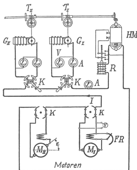
Fig. 15 Schaltplan einer Gleichstromanlage nach Thury [A2]
