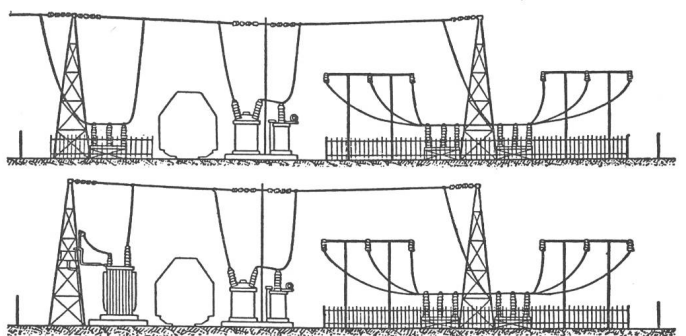
Fig. 7 Freiluftanlage in Flachbauweise (Sachsenwerk) [A 4]
