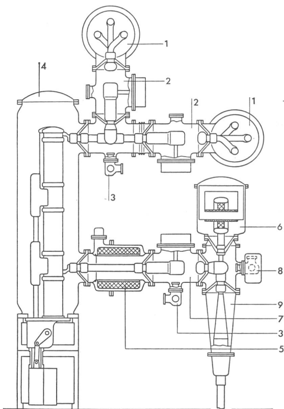
Fig. 14 Schnitt durch ein SF 6 -Schaltfeld mit Doppelsammelschienen (BBC) [B6]
