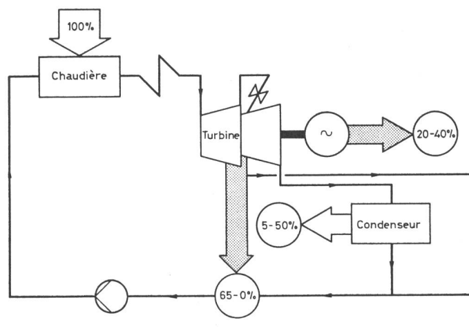
Fig. 5 Installation à vapeur: condensation avec soutirage
