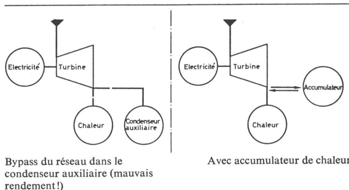
Fig. 4 Amélioration de la flexibilité d'une centrale à contre-pression
