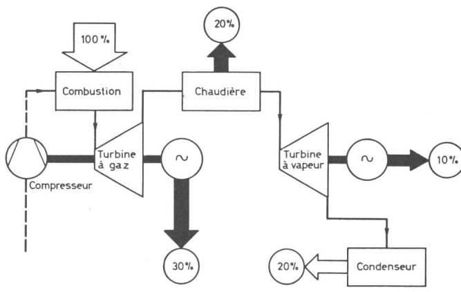
Fig. 9 Combinaison turbine à gaz/turbine à vapeur
