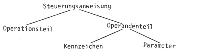
Fig. 4 Aufbau der Steuerungsanweisung nach DIN-Entwurf
