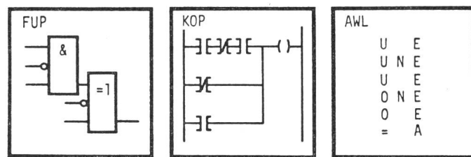
Fig. 5 Übersicht der Programmiersprache STEP 5
