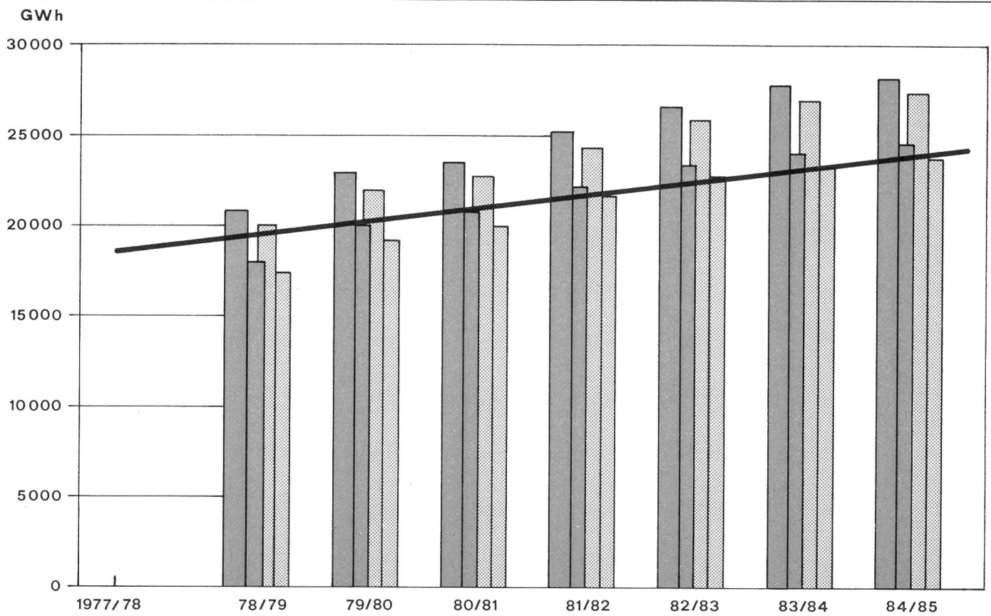
Fig. 7 Vergleich des mutmasslichen Verbrauchs und der voraussichtlichen Erzeugungsmöglichkeiten im Winter unter verschiedenen Randbedingungen
