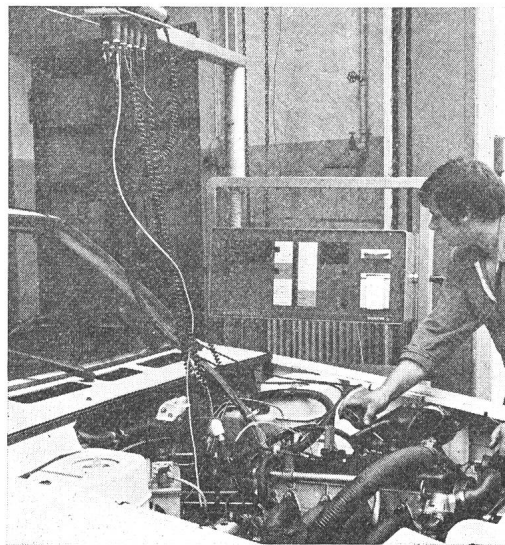
Fig. 6 Motortester 631
