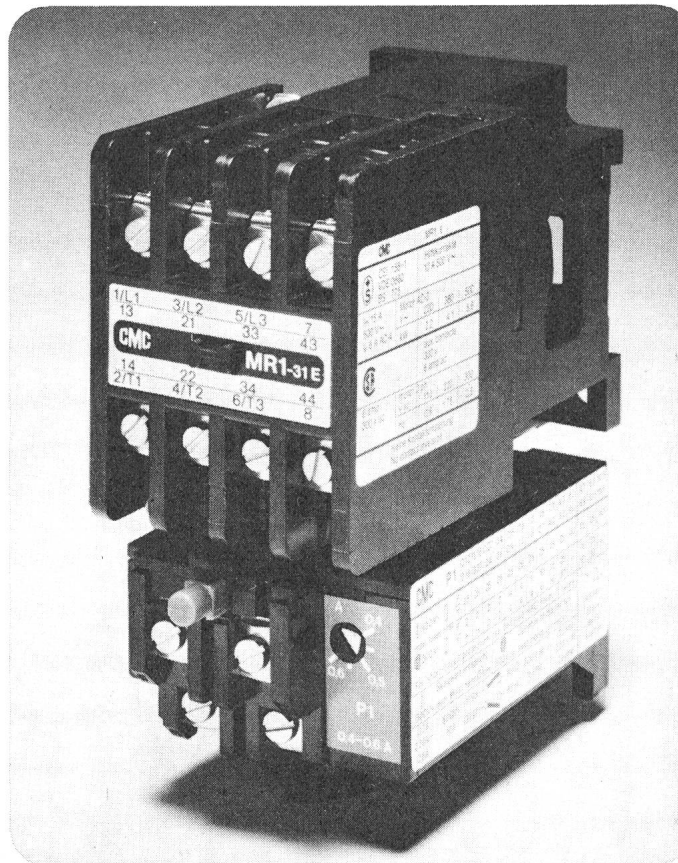
MR1PE, Klein-Motorschütz nach Euronorm
