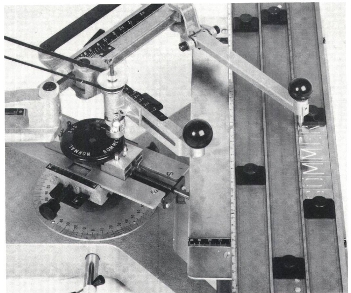
Gravieren auf einem unebenen Schalterring in Kreisanordnung
