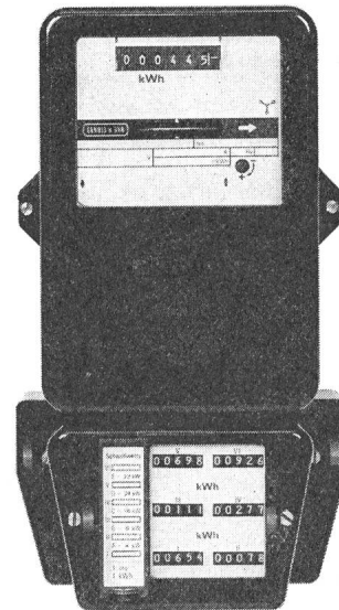
Leistungsabhängige Energiemessung mit Stufeneinteilung
