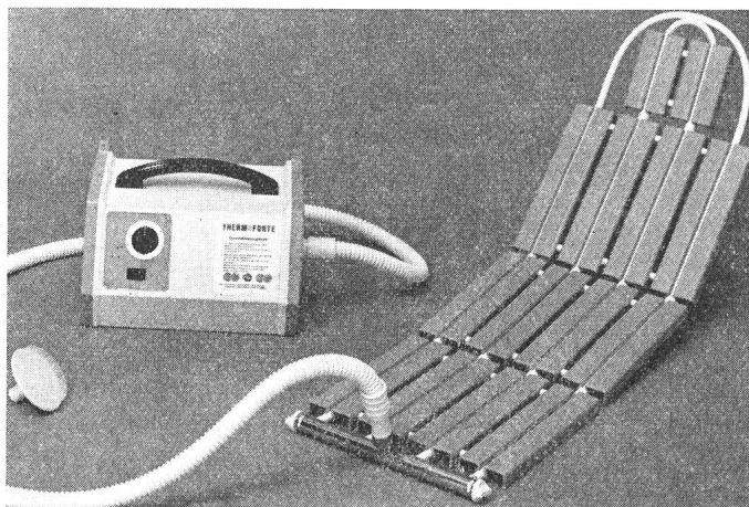
Luftsprudelbad Thermofonte
