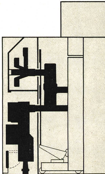
Metallgeschützte und geschottete Bauart (Typ PEDC)
