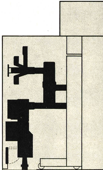
Metallgeschützte Bauart (Typ PEC)
