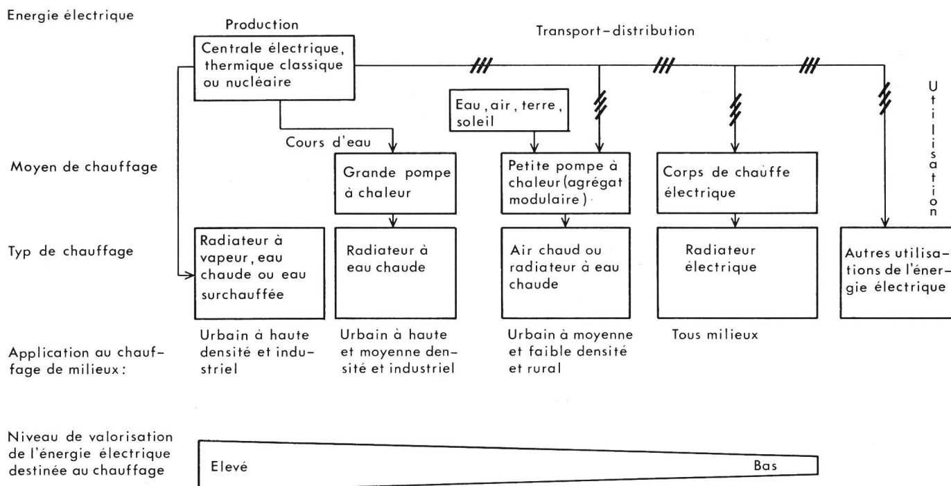
Fig. 1 La place de la pompe à chaleur modulaire dans le système intégré, centrale et réseau électriques force-chaleur
