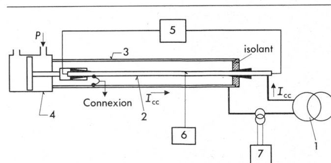
Fig. 6 Installation d'essai
