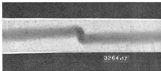
Fig. 8 Déformation de la cordelette HF de la paire coaxiale après essais de court-circuit de l'échantillon n° 3 (tableau IV), photographie prise par transparence
