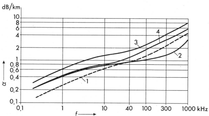
Fig. 2 Affaiblissement linéique \alpha en fonction de la fréquence f
