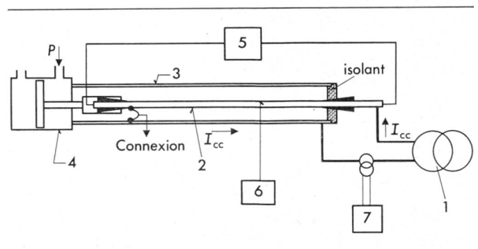
Fig. 6 Installation d'essai
