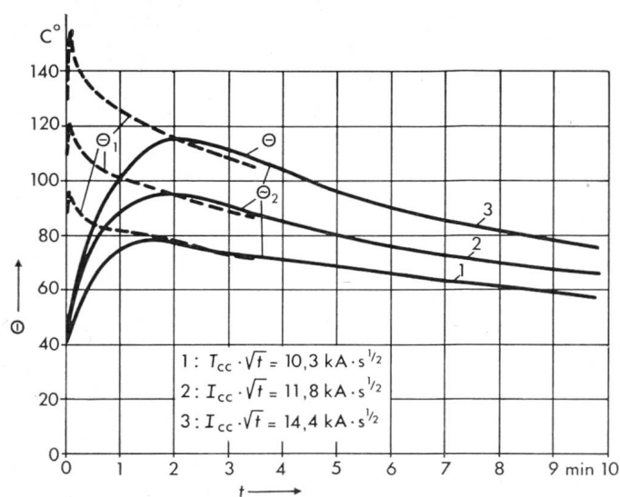
Fig. 7 Variation de la température \Theta dès la fin du court-circuit pour le câble de garde avec paire coaxiale, câble n° 1 (Aldrey/Alumoweld: 100/50 mm 2 )
