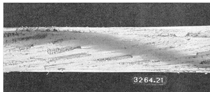
Fig. 9 Déformation de la cordelette HF de la paire coaxiale après essais de court-circuit de l'échantillon n° 4 (tableau IV), photographie prise par transparence
