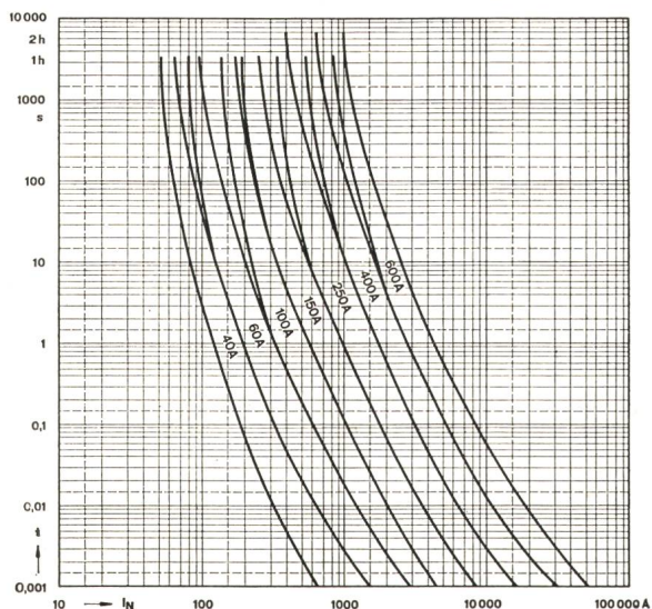
Schmelzleiter und Abschmelzcharakteristik Trägheitsgrad 2/1
