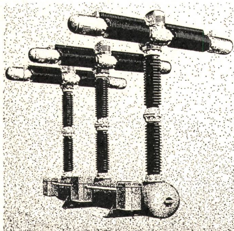
Druckluftschalter
