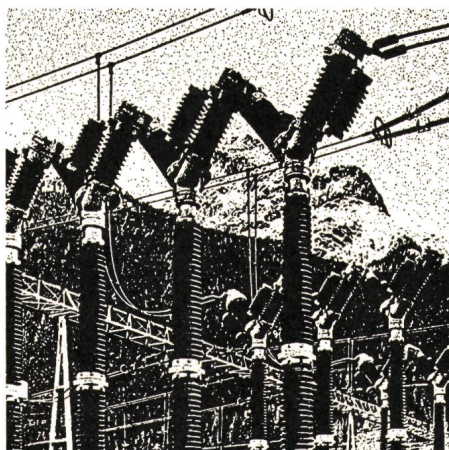
Oelarme Schalter
