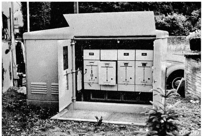
Fig. 6 Minikabine Peyer mit 18 kV «Krone»-Zelle
