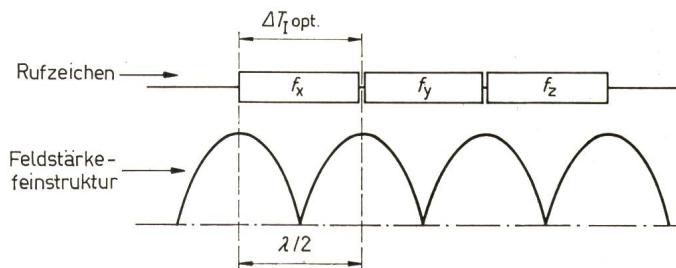
Fig. 3 Feldstärkefeinstruktur und optimale Impuls-Zeichenlänge \Delta T_{\text{I opt.}} optimale Impulslänge; f_x, f_y, f_z Codefrequenzen; \lambda HF-Wellenlänge
